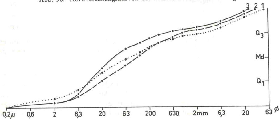
Abb. 31. Kornsummenkurven der Bunten Breccie von Otting.
